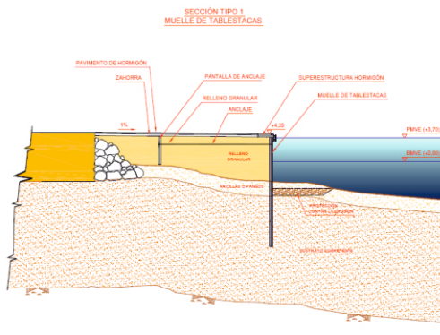
Secciones Tipo
