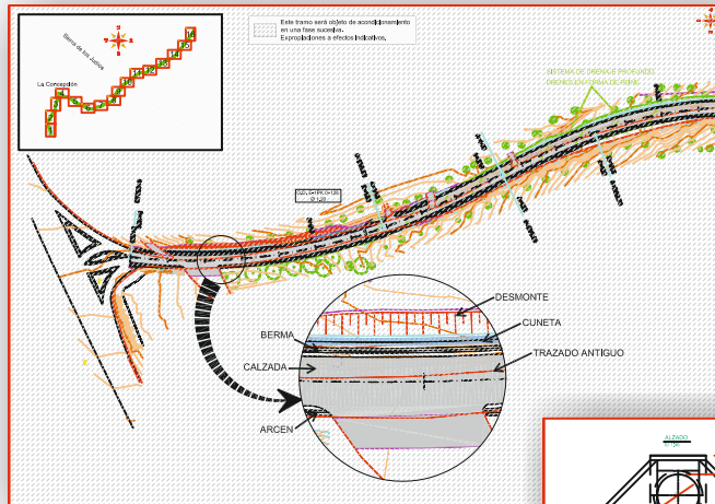
Planta de trazado
