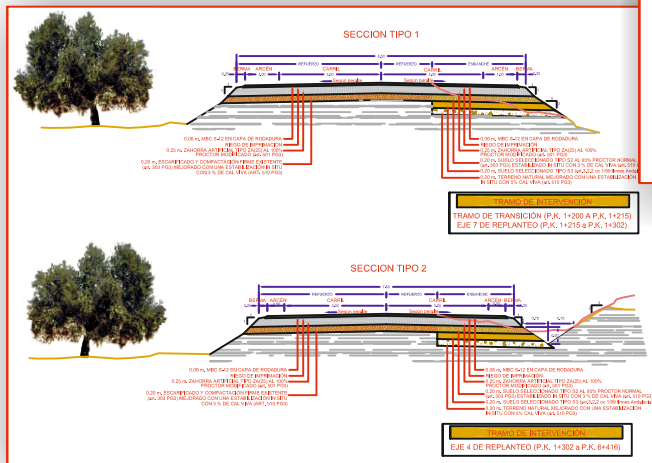
Secciones tipo
