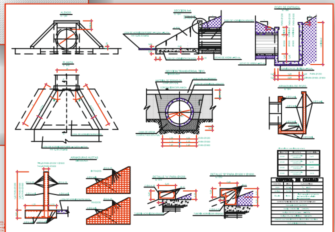
Detalles de drenaje
