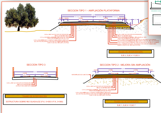
Sección tipo
